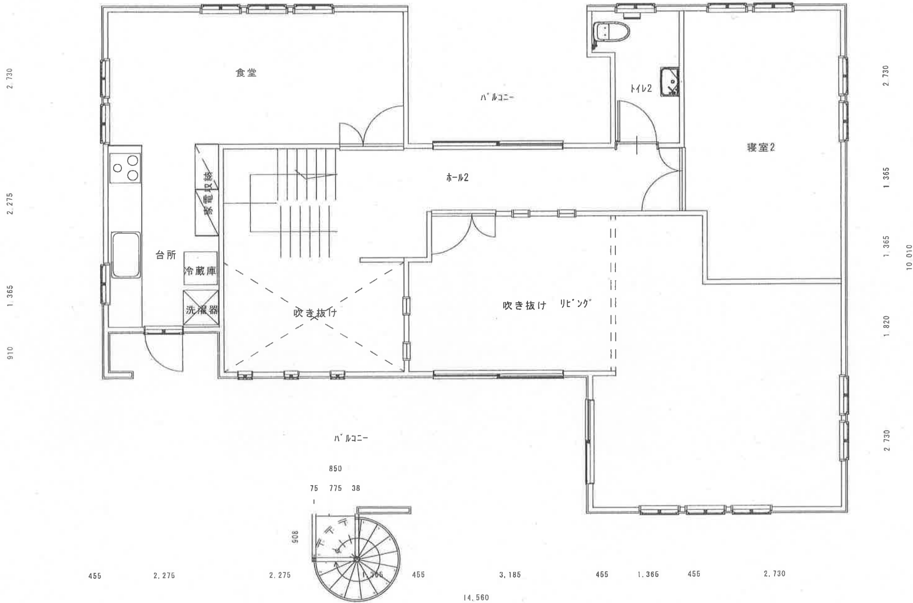
2 階平面図
