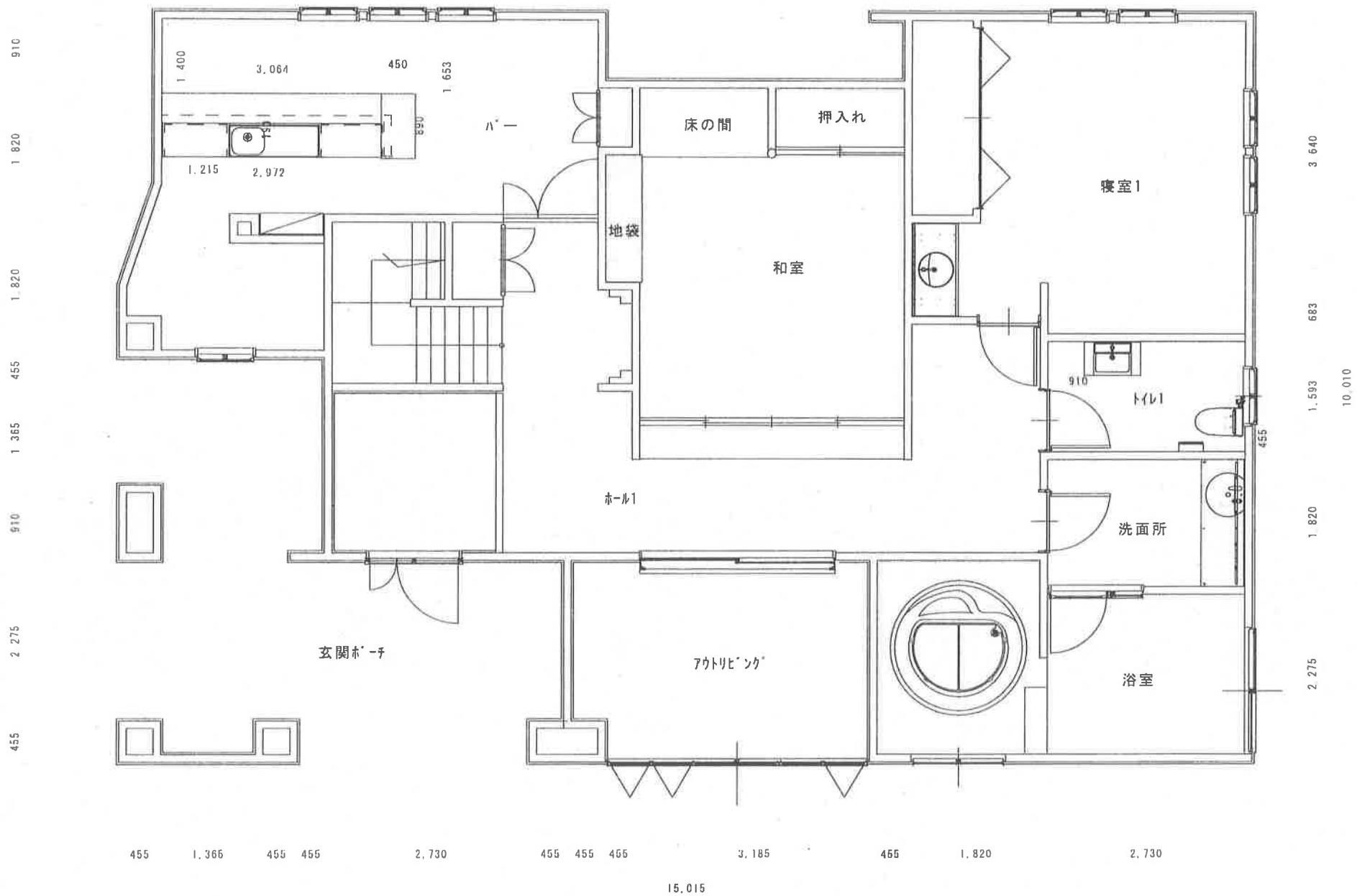
1 階平面図
