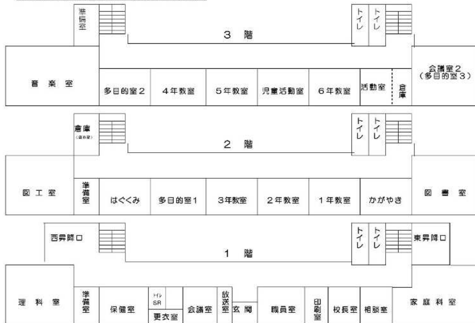
令和6年度日川小学校教室配置図
