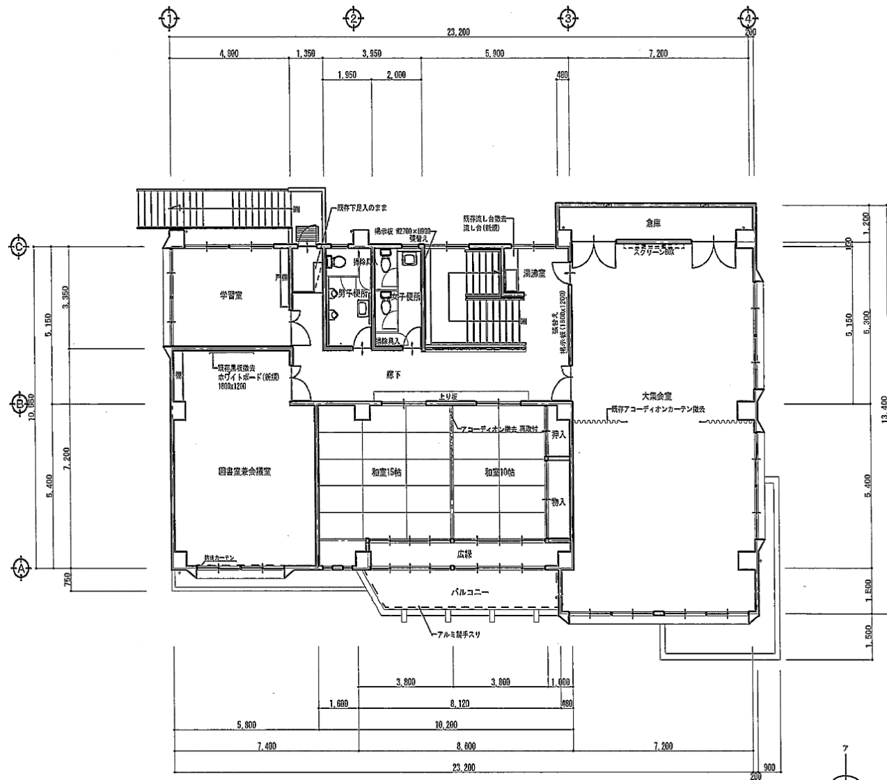
補強後 2階平面図 S=1/100
