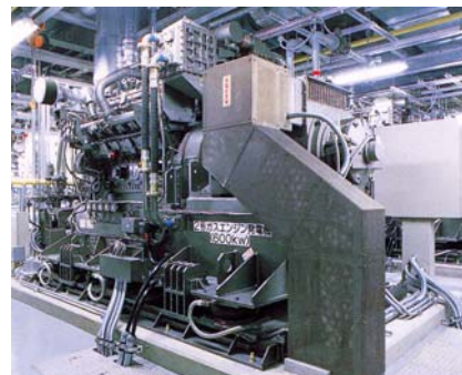
天然ガスコージェネレーション (ガスエンジン) (都立豊島病院(東京都))
