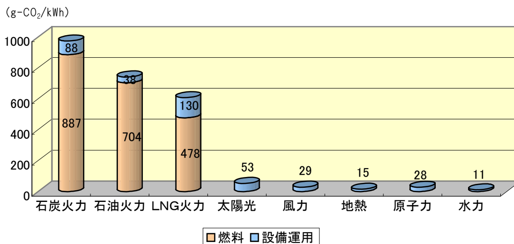
図 2.2-2 日本における電源別の二酸化炭素排出量
