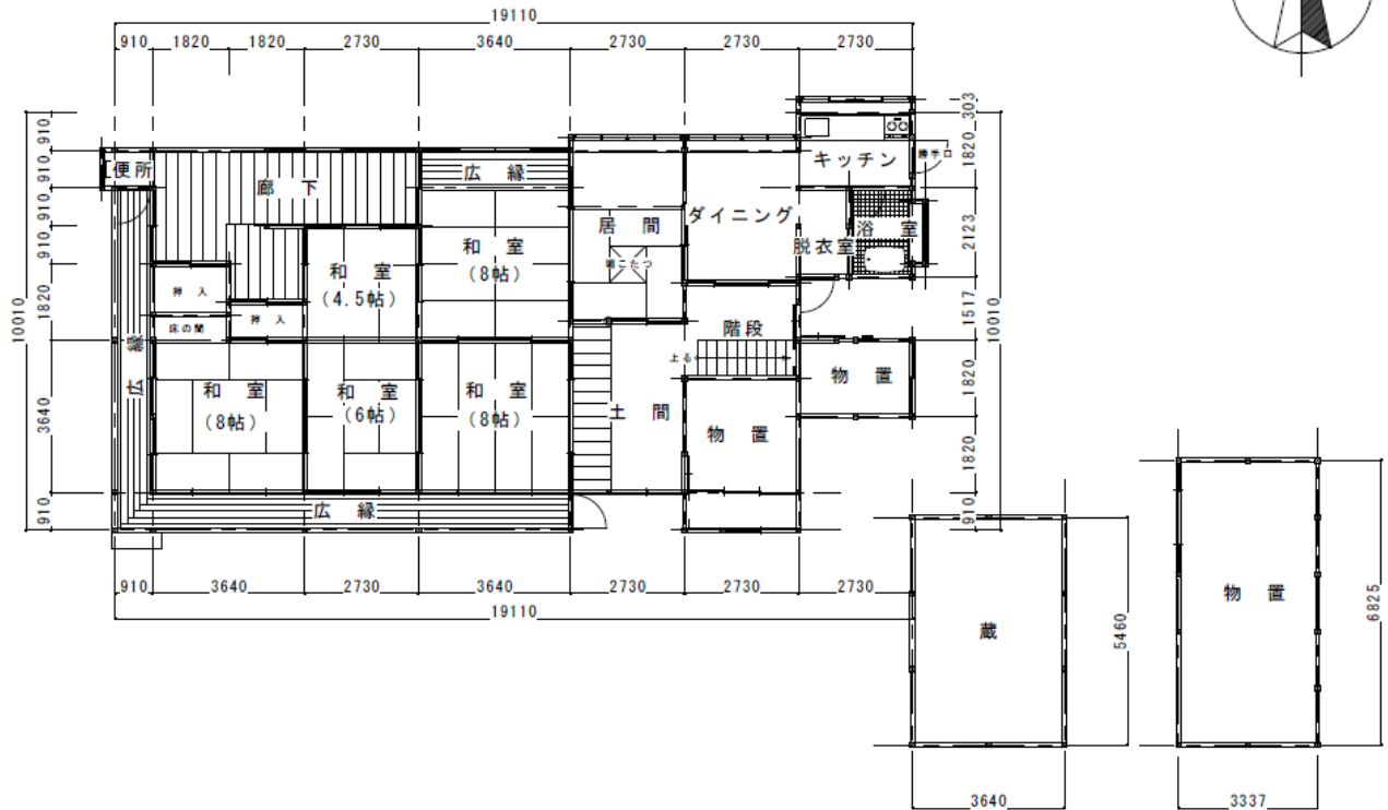
1階 縮尺 1/150
