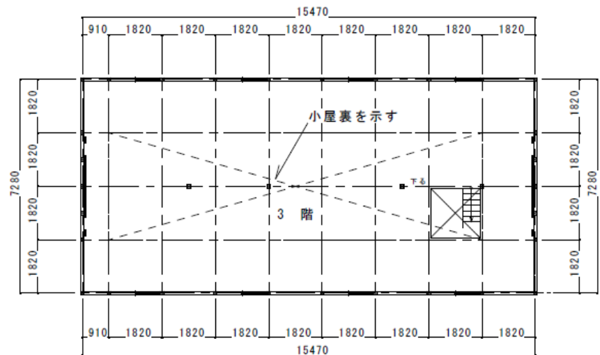
3階 縮尺 1/150
