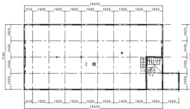
2階 縮尺 1/150
